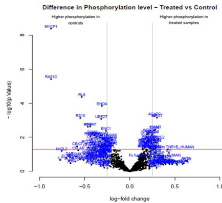
リン酸化レベルのボルケーノプロット
